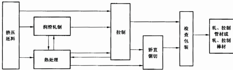
图 1 轧、控制管材和轧、控制棒材生产工艺流程简图
